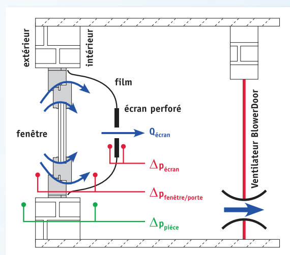
Principe pour la détermination de la perméabilité des fenêtres
